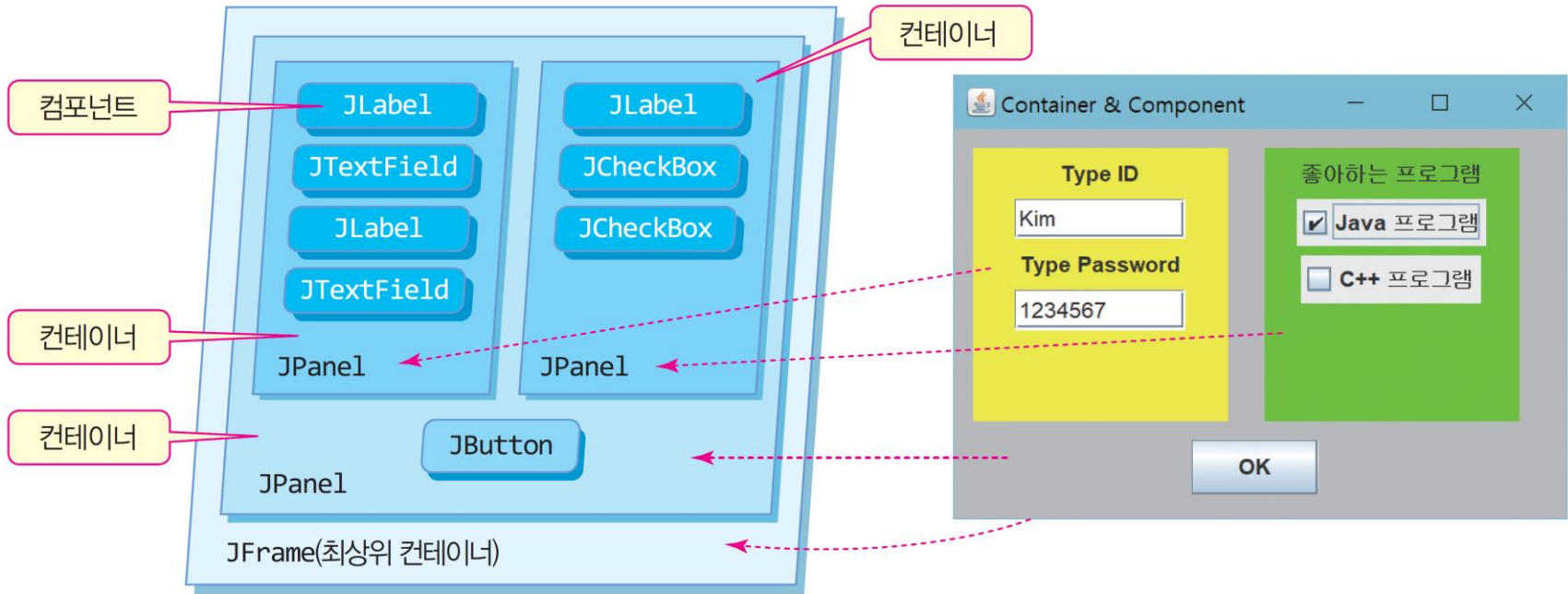
스윙 컨테이너와 컴포넌트의 포함 관계
