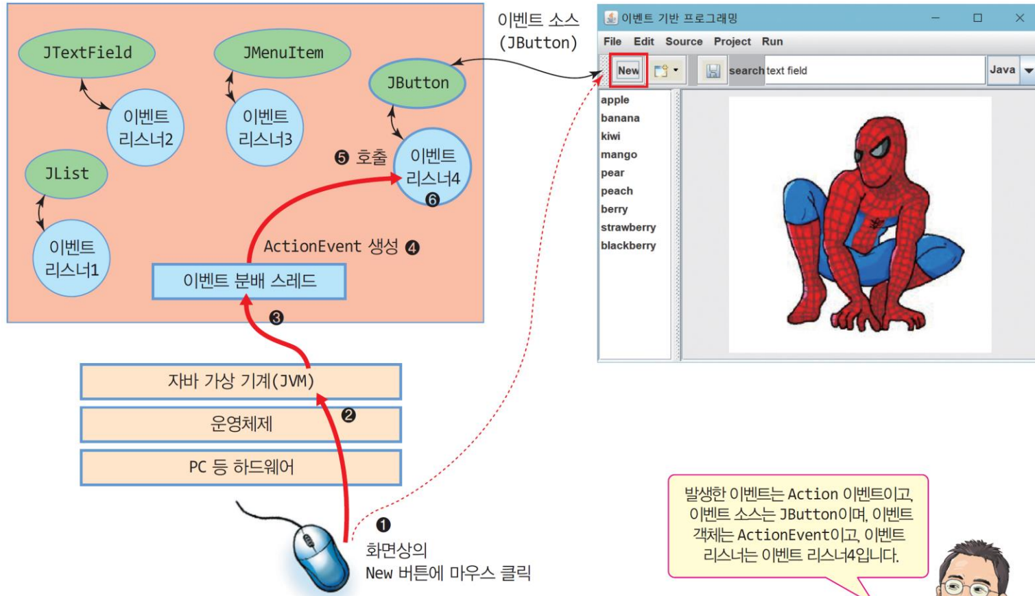
자바 응용프로그램
